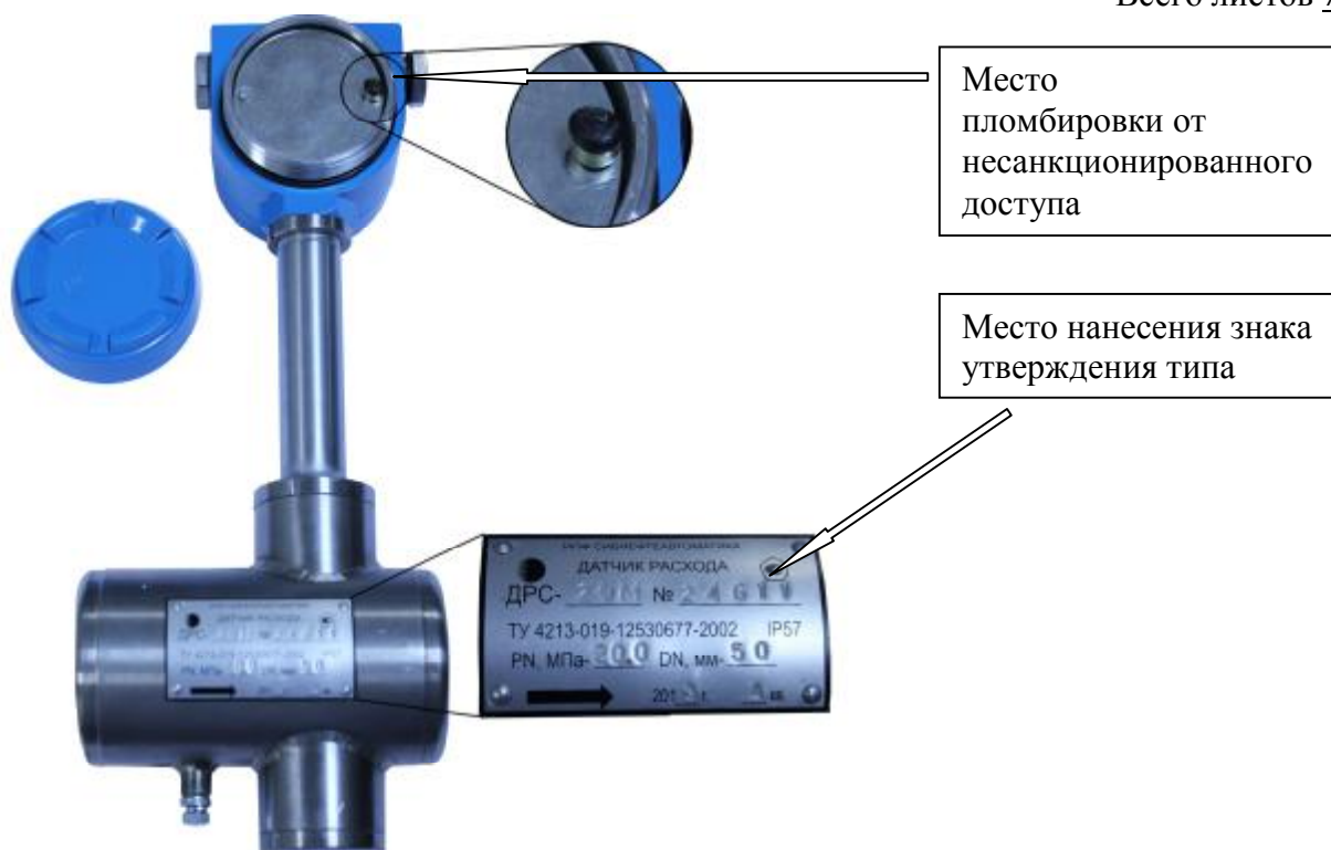
Рисунок 1. Датчика расхода ДРС
